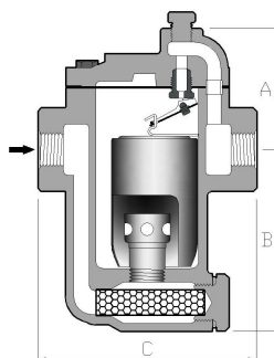
No.980 系列 尺寸單位 (MM). 重量 (KG)
